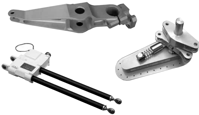
航空機に搭載される部品
