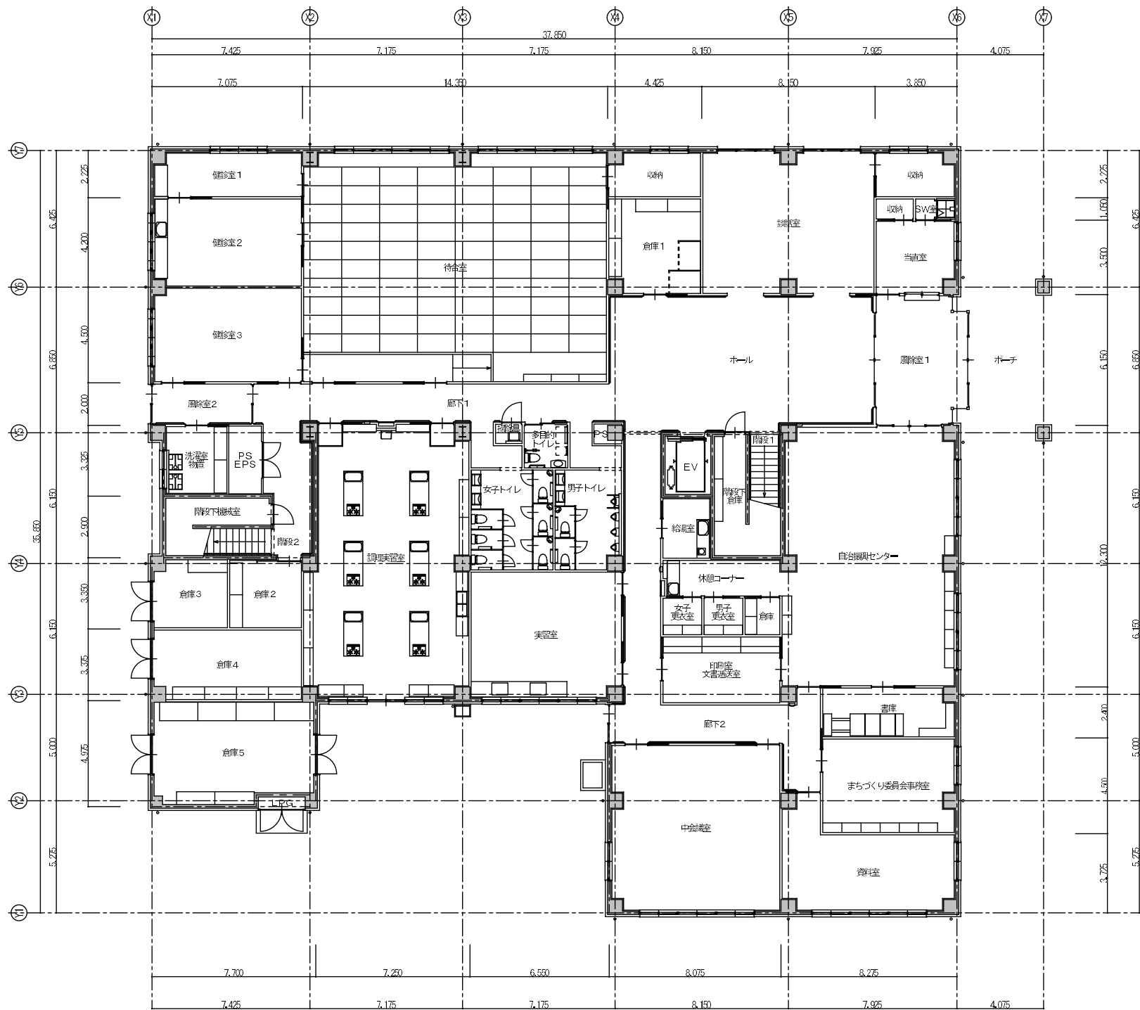
1階平面図 1/100
