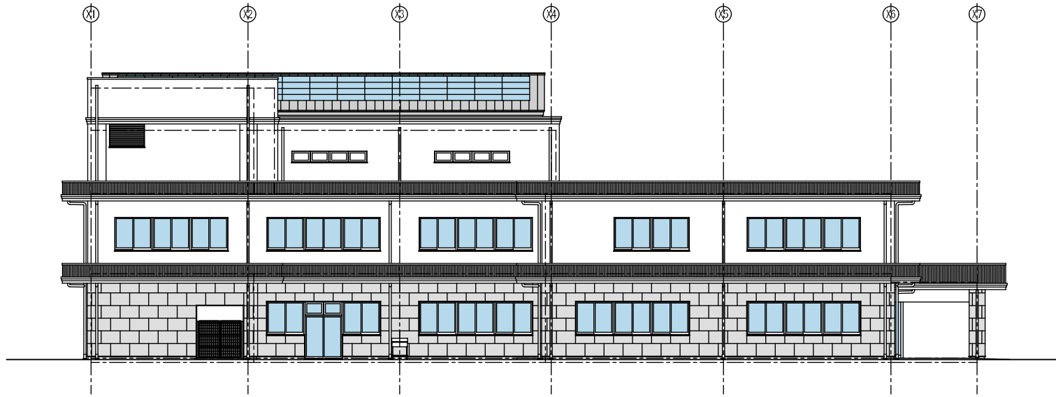
南側立面图 1/100
