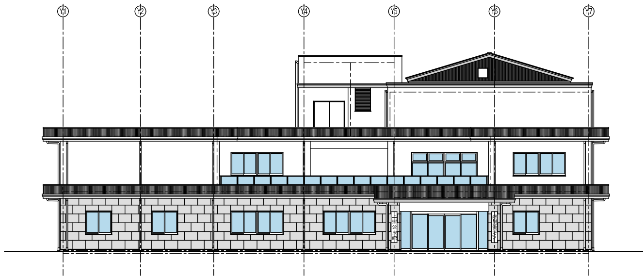
東側立面图 1/100
