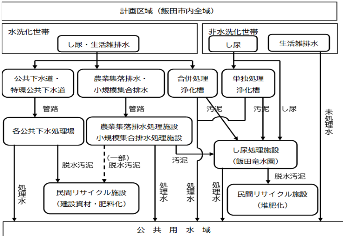
図1 処理体系図
