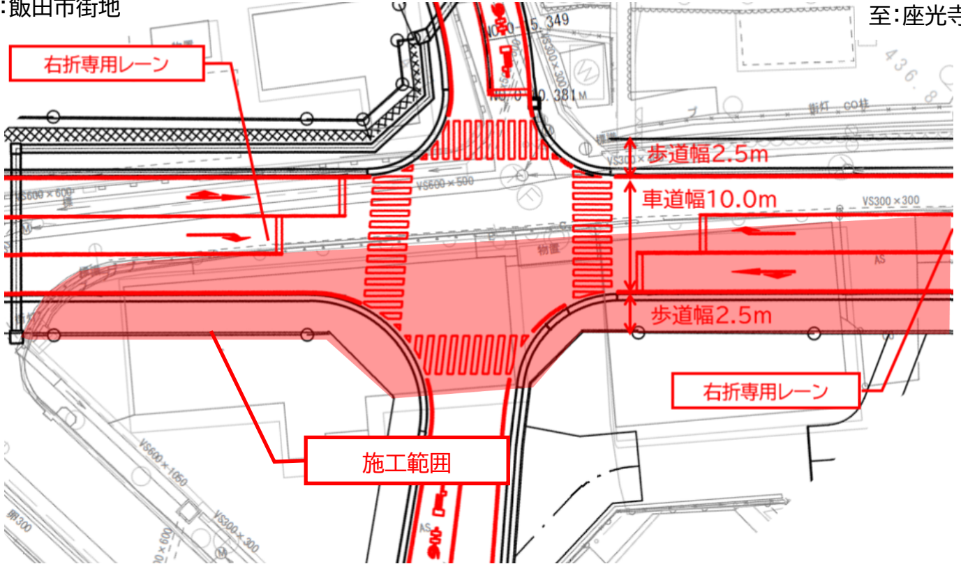
平面図
