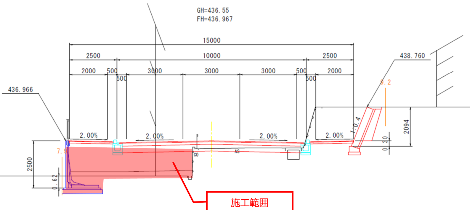
横断面図
