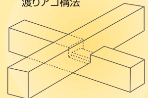
渡りアゴ構法
