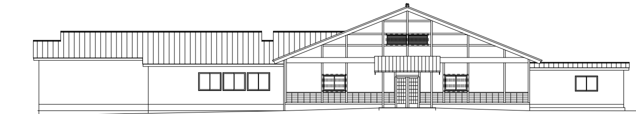
西側立面図
