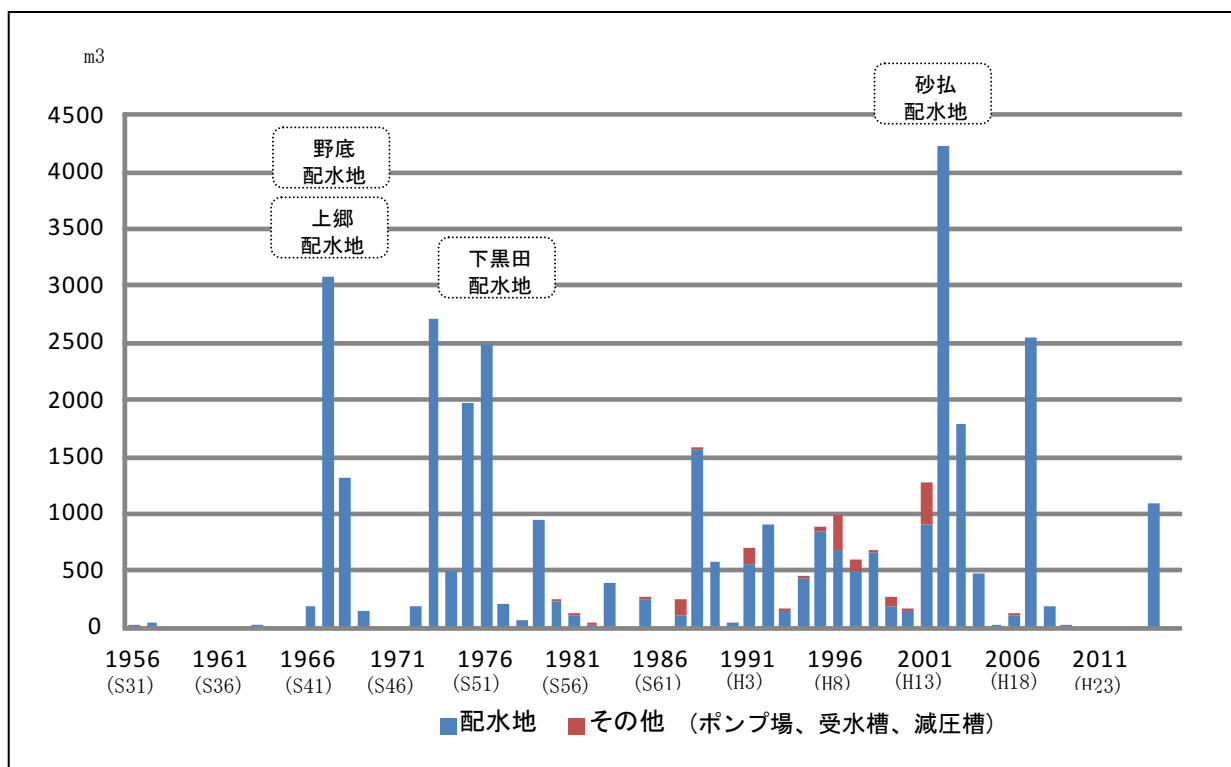
【 上水道施設(浄水場以外の施設)の年度別整備容量 】
