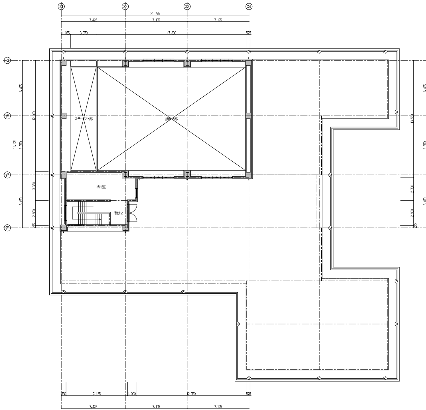
PH階平面図 1/100
