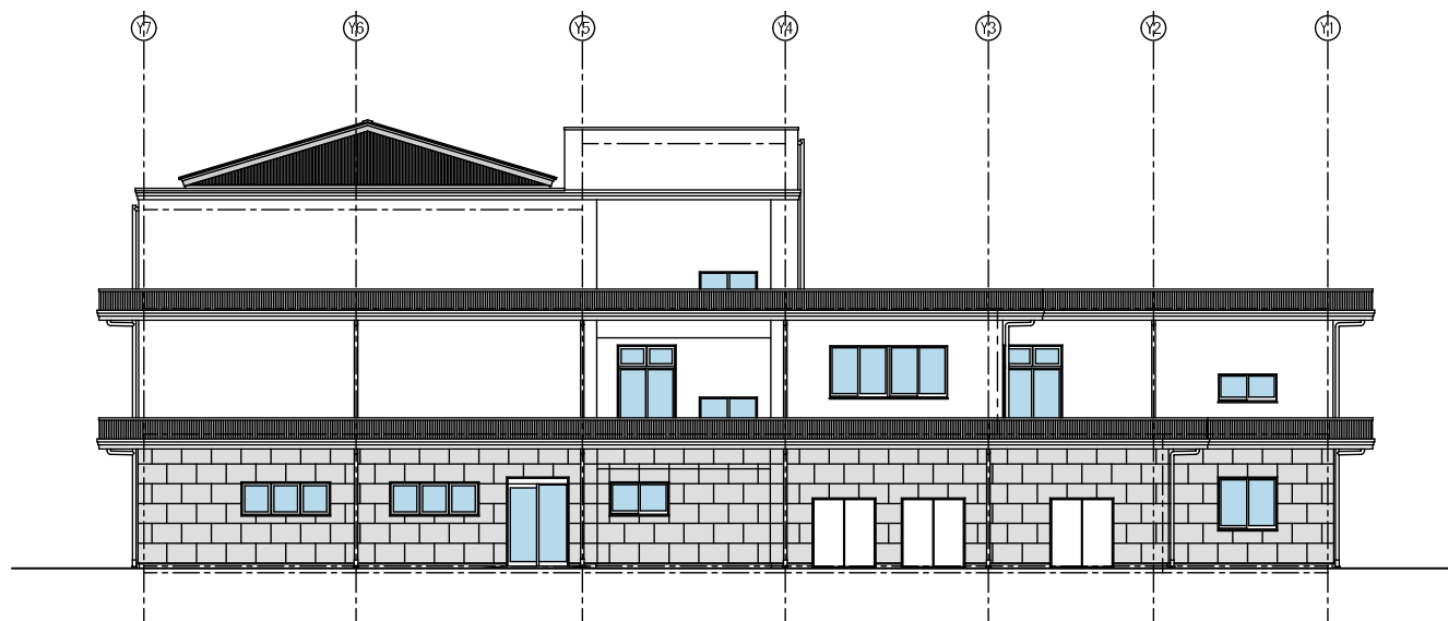
西側立面図 1/100
