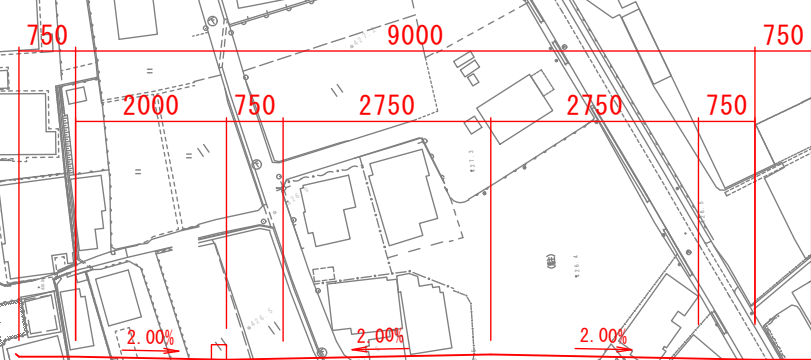
市道上郷489号線 標準横断面図
