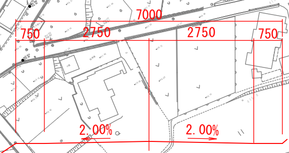
市道上郷490号線 標準横断面図
