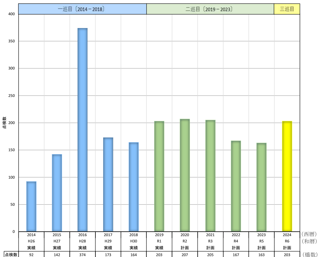
図 4-1 定期点検実施道路橋数（実績・計画）
