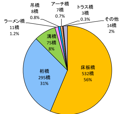
図 2-2 構造形式別の道路橋数
