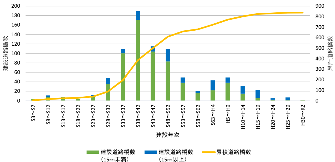
図 2-3 道路橋の建設年別分布（基準年：令和 2 年 3 月末時点）
