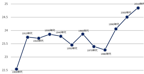
7月平均気温 2.31°C上昇
