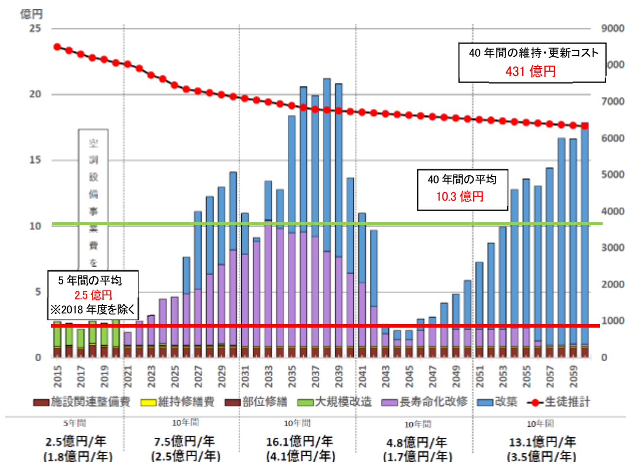
図 長寿命化形改修と計画的改修によるコスト試算
