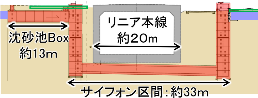
断面図
