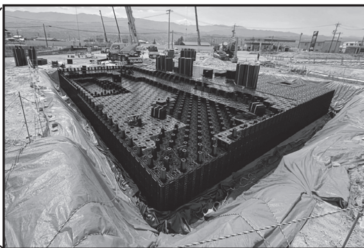
北側調整池整備工事(令和7年6月)
