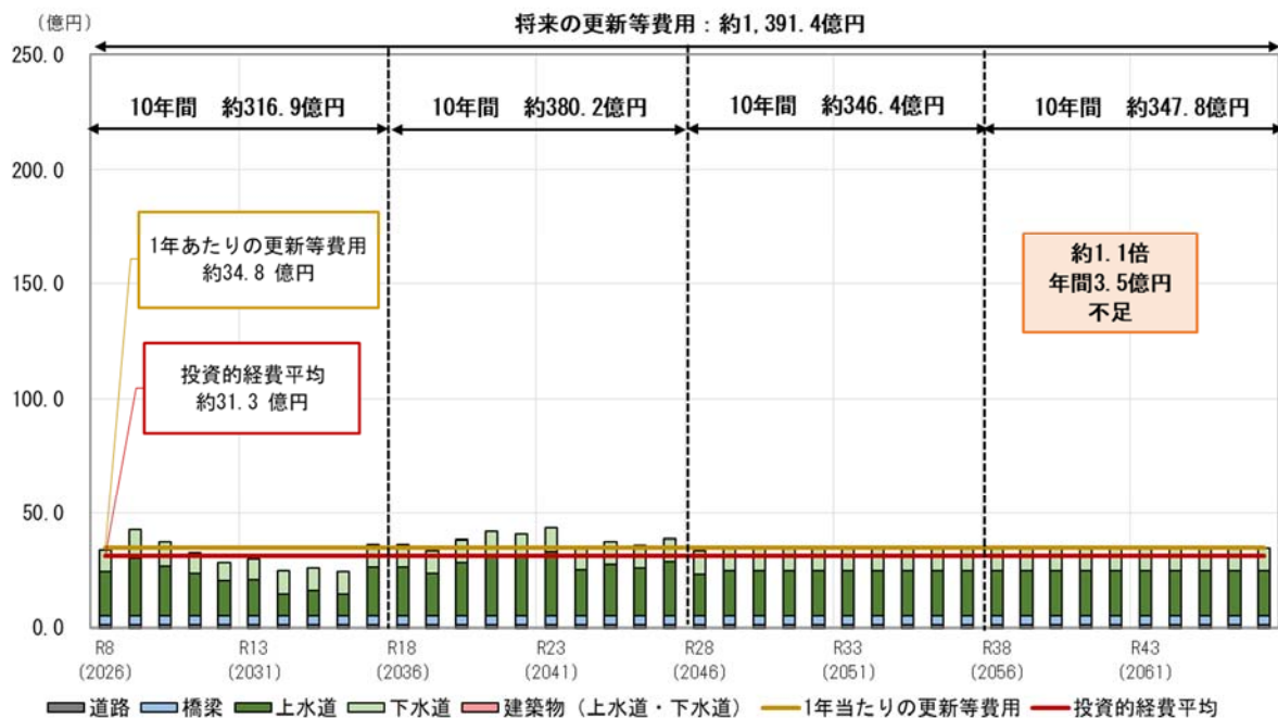
図 インフラ施設の将来の更新等費用の推計（対策後費用）
