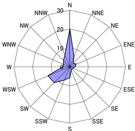
風配図
