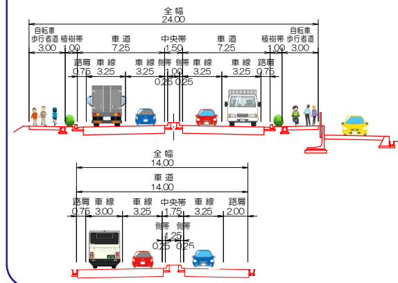
座光寺上郷道路 標準横断面図
