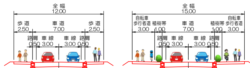
東新町座光寺線 標準横断図
