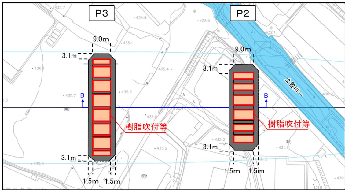
ケーソン基礎（P 2， P 3）平面図
