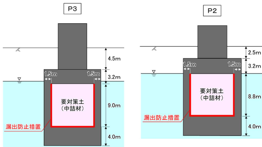
ケーソン基礎（P 2， P 3）断面図（B－B断面）
