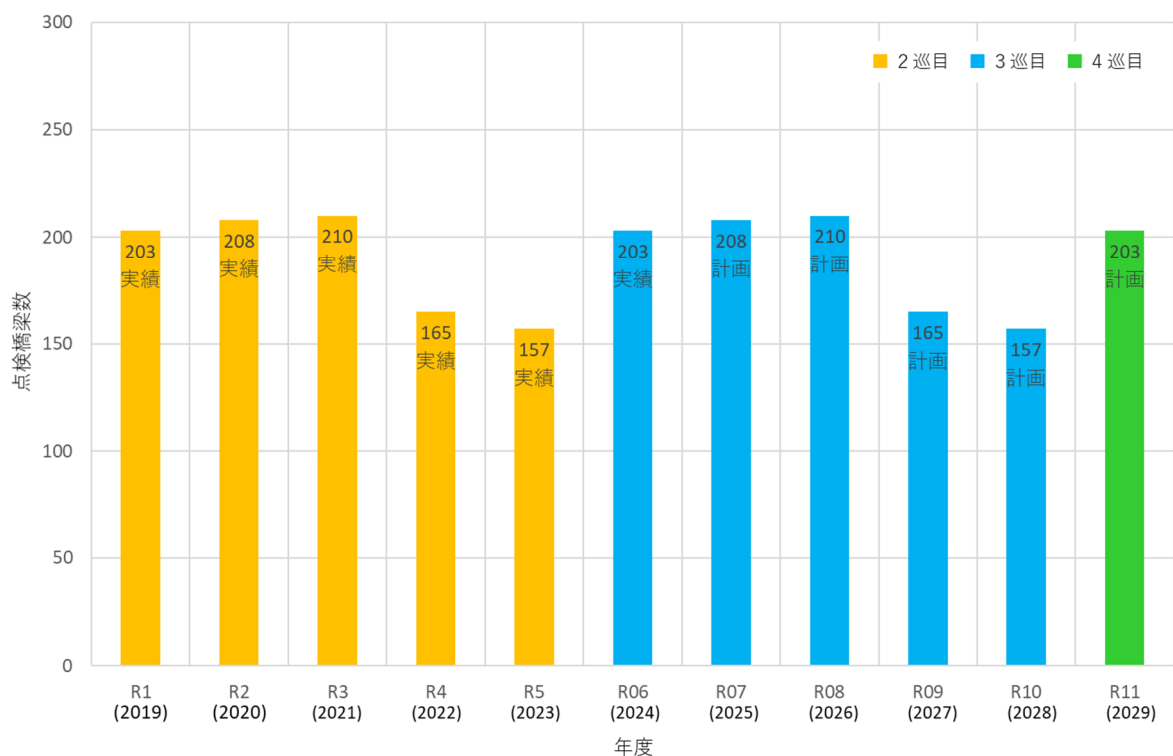
図 4-1 定期点検実施道路橋数（実績・計画）
