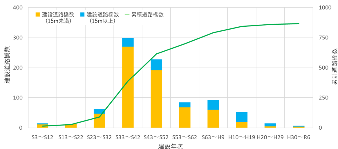
図 2-3 道路橋の建設年別分布（基準年：令和 6 年 3 月末時点）
